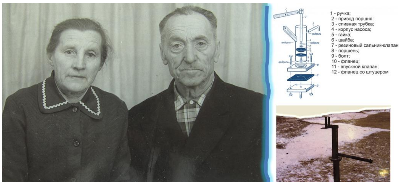
Рис. Пет-08. Слева: Екатерина Ивановна и Яков Абрамович Петкау в зрелые годы жизни. Справа: Остов колонки конструкции «Петкау» – безмолвный памятник «Главному специалисту» по водоснабжению в Прииск-Кумаке, Комарово и их окрестностях
