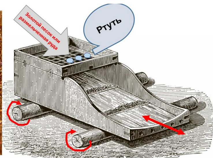
Рис. ТДЗ-01. Слева: так выглядит кварцевый песок с частичками золота. Справа: вашгерд (производное слово от немецких: waschen – мыть и Herd – плита) – оборудование с возвратно-поступательным столом (плитой) для промывки золотого песка или размельченной руды. Сюда же добавлялась ртуть для отделения золота от породы
