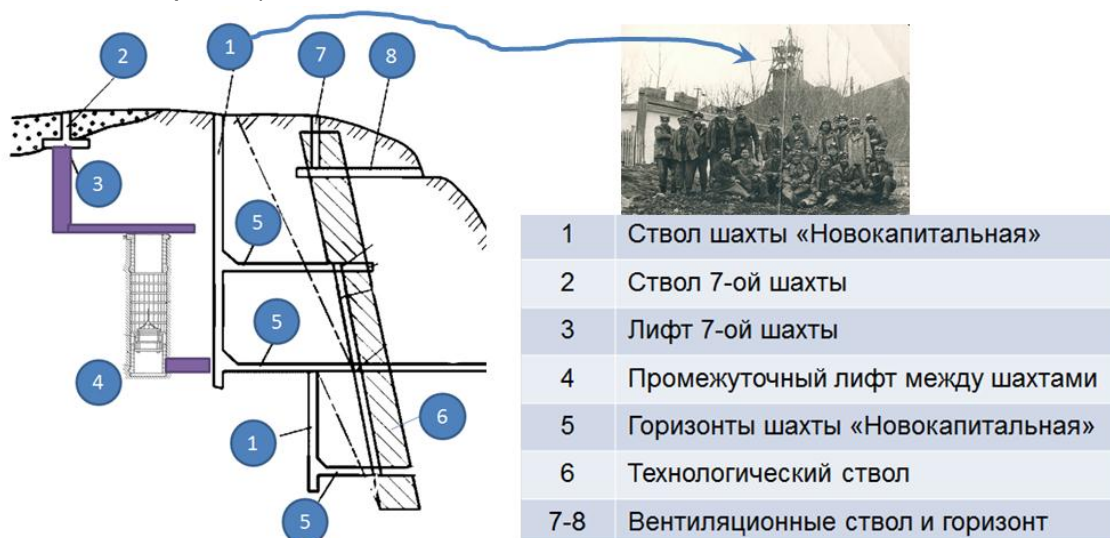
Рис. ИГМ-03. Условная схема соединения шахт рудника Кумаг, составлена автором по рассказам нескольких очевидцев
